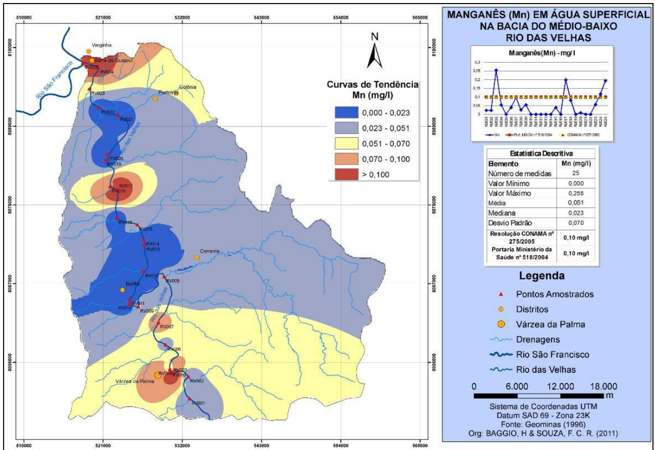
Figura 8 - mapa de isotores apresentando a distribuição espacial do Mn total, ao longo do baixo curso do Rio das Velhas
