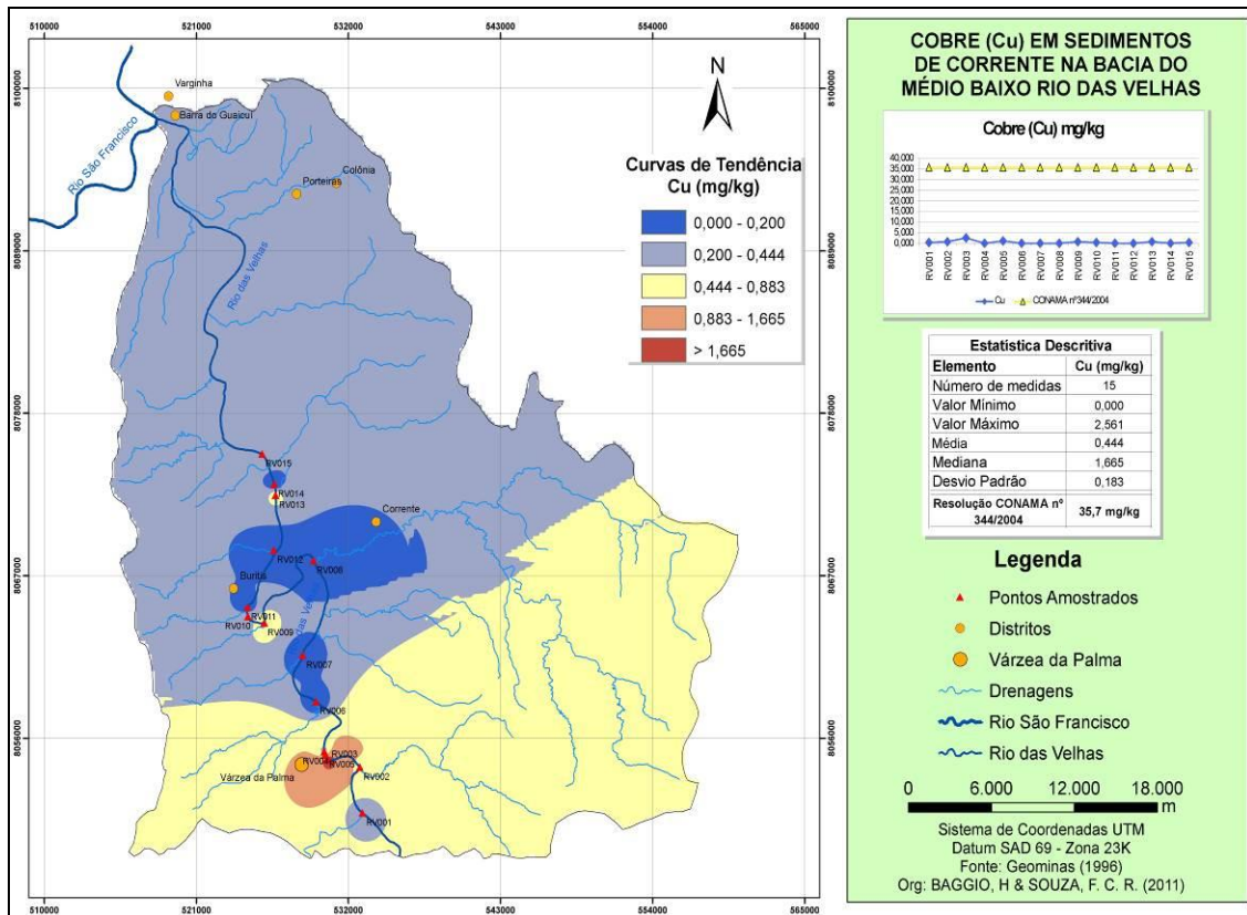
Figura 9 - mapa de isotores apresentando a distribuição espacial do Cu total, ao longo do baixo curso do rio das Velhas
