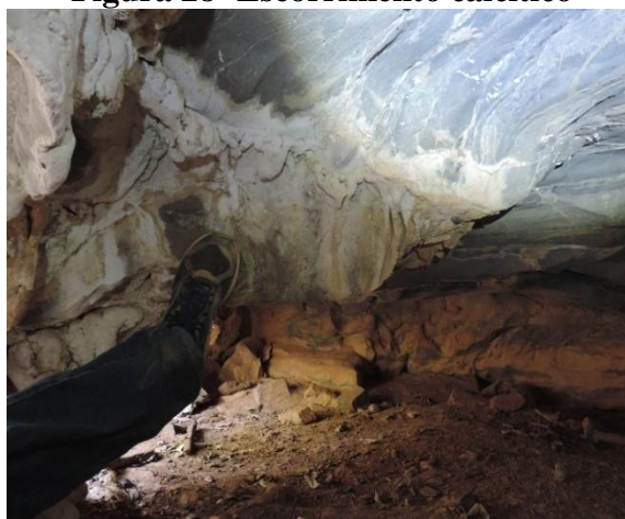
Figura 28- Escorrimento calcítico
