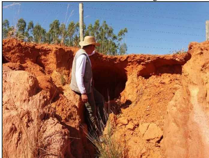
Figura 9 - Processo erosivo no horizonte B - Argissolo Vermelho
