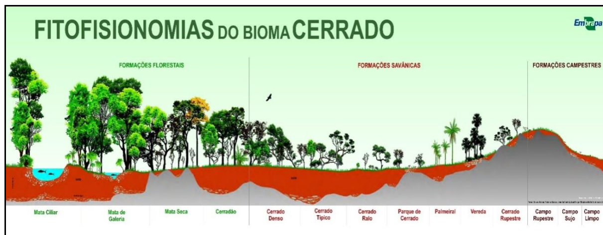
Figura 1 – Perfil esquemático das fitofisionomias do bioma Cerrado
