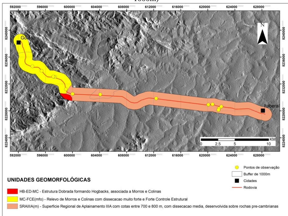
Figura 4 – Mapa de Unidades Geomorfológicas das margens da rodovia GO-070 (buffer de 1000m)
