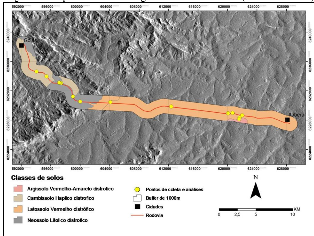
Figura 3 – Mapa de solos das margens da rodovia GO-070 (buffer de 1000m)
