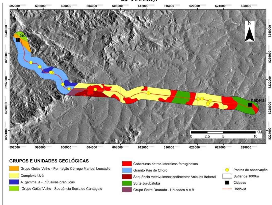
Figura 5 – Mapa de Grupos e Unidades Geológicas das margens da rodovia GO-070 (buffer de 1000m).
