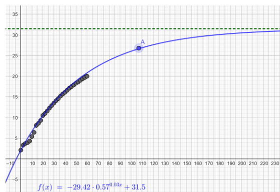
Figura 7: Uma proposta de modelo aproximado para o aquecimento do líquido analisado (Elaboração própria)
