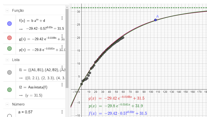
Figura 9: Comparação gráfica entre as três funções encontradas para o comportamento térmico analisado (Elaboração própria)
