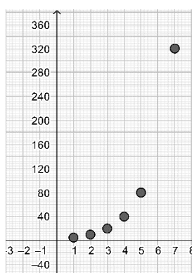
Figura 2: Projeção dos pontos que associam a quantidade de vitórias-régias em função dos dias (Elaboração própria)
