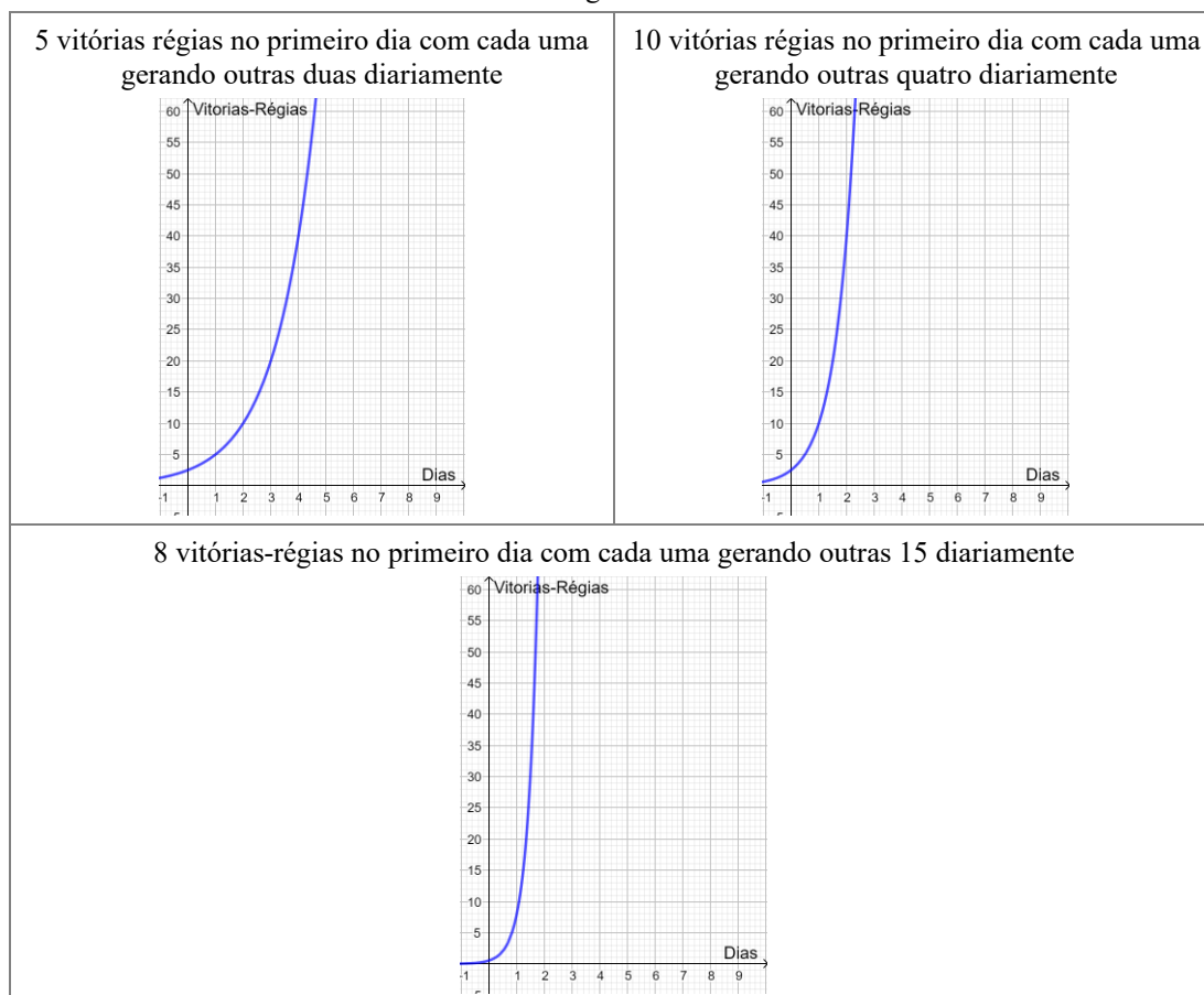
Quadro 6: Análise gráfica da variação das unidades significativas da função exponencial sem sua representação em língua natural
